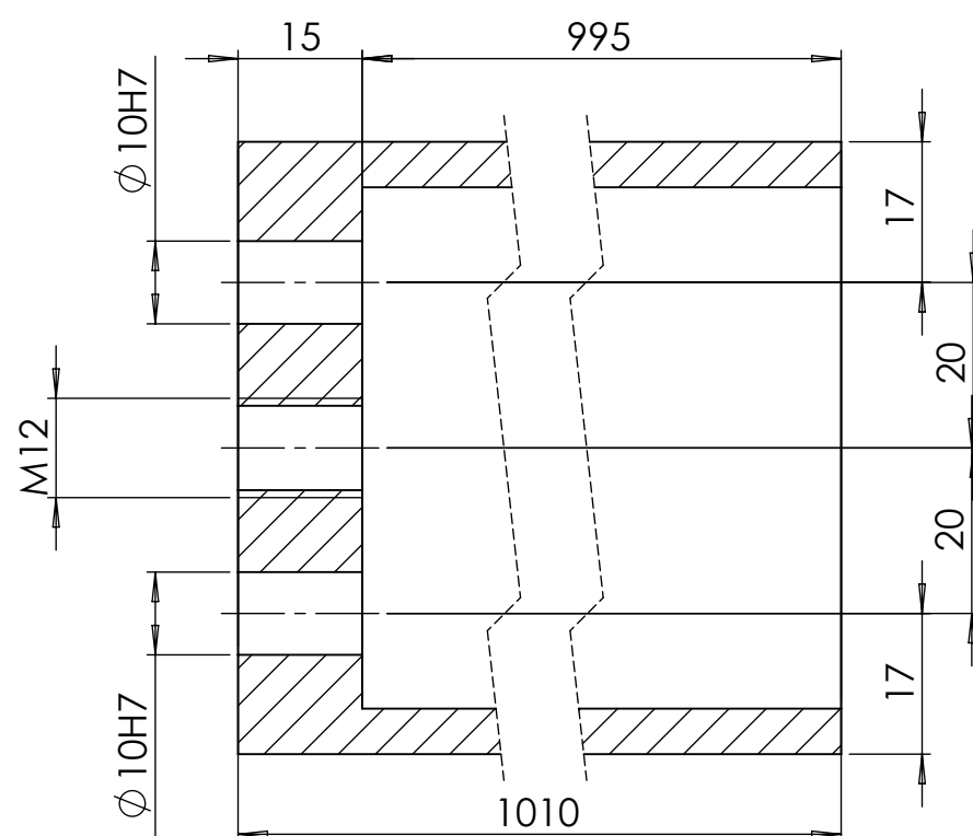
ŘEZ A-A MĚŘÍTKO 1 : 1
