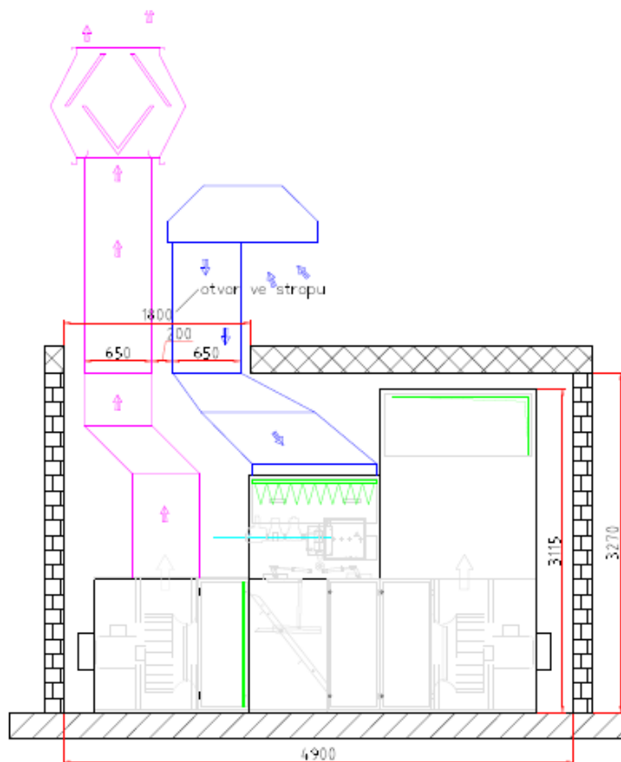
boční pohled na agregát kabiny - pohled od dveří do strojovny
